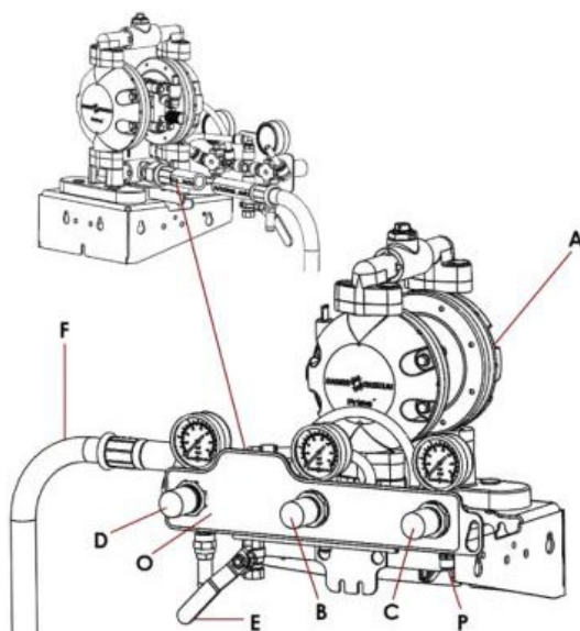
Wizualizacja z pompą 01D100 wyposażoną w 3 regulatory powietrza
